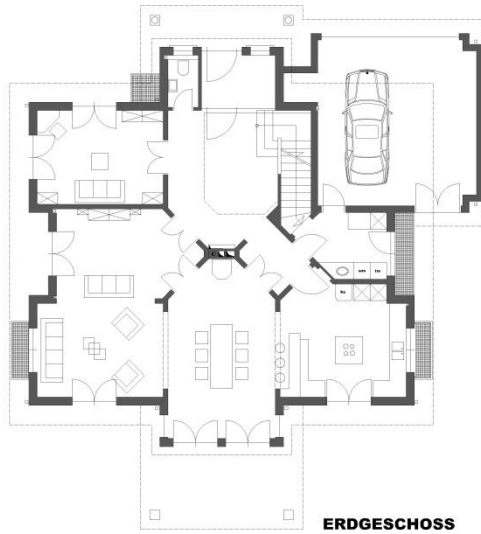
ERDGESCHOSS
